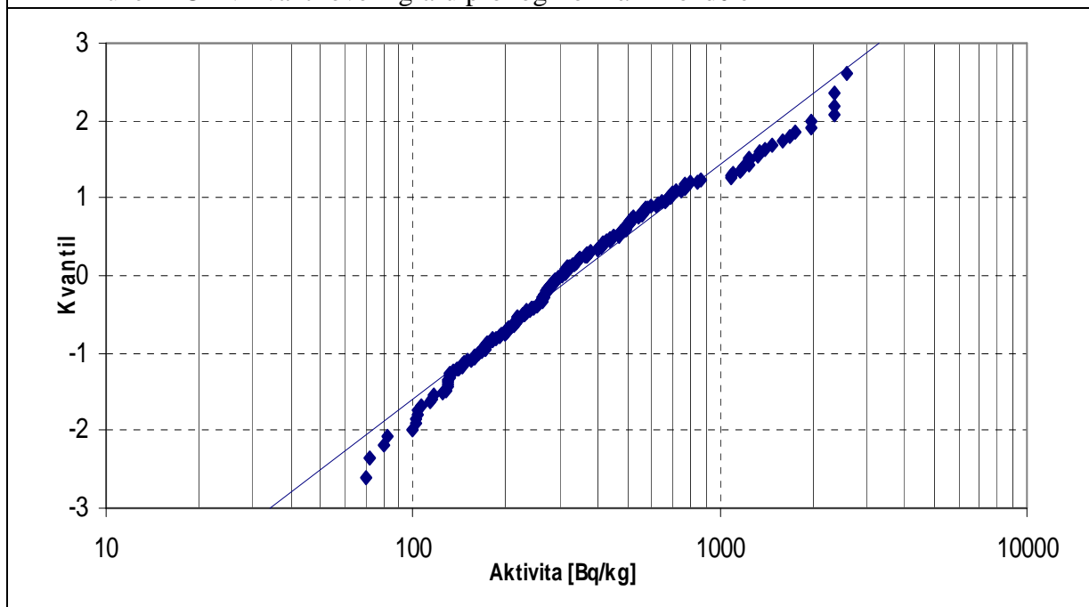
Obr 2 Hmotnostní aktivita ^{137}\text{Cs} v humusech odebraných v roce 1995 odebraných na území ČR v kvantilovém grafu pro log-normální rozdělení
