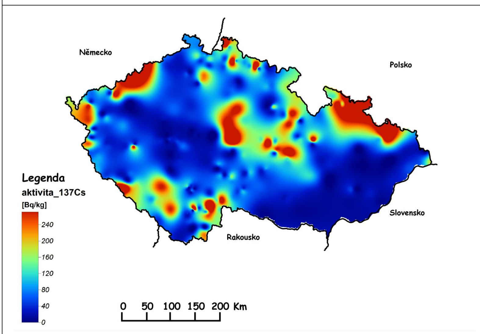
Obr. 1b Hmotnostní aktivity ^{137}\text{Cs} v hřibotvarých houbách na území ČR v letech 2004 – 2012 – vyhlazené zobrazení
