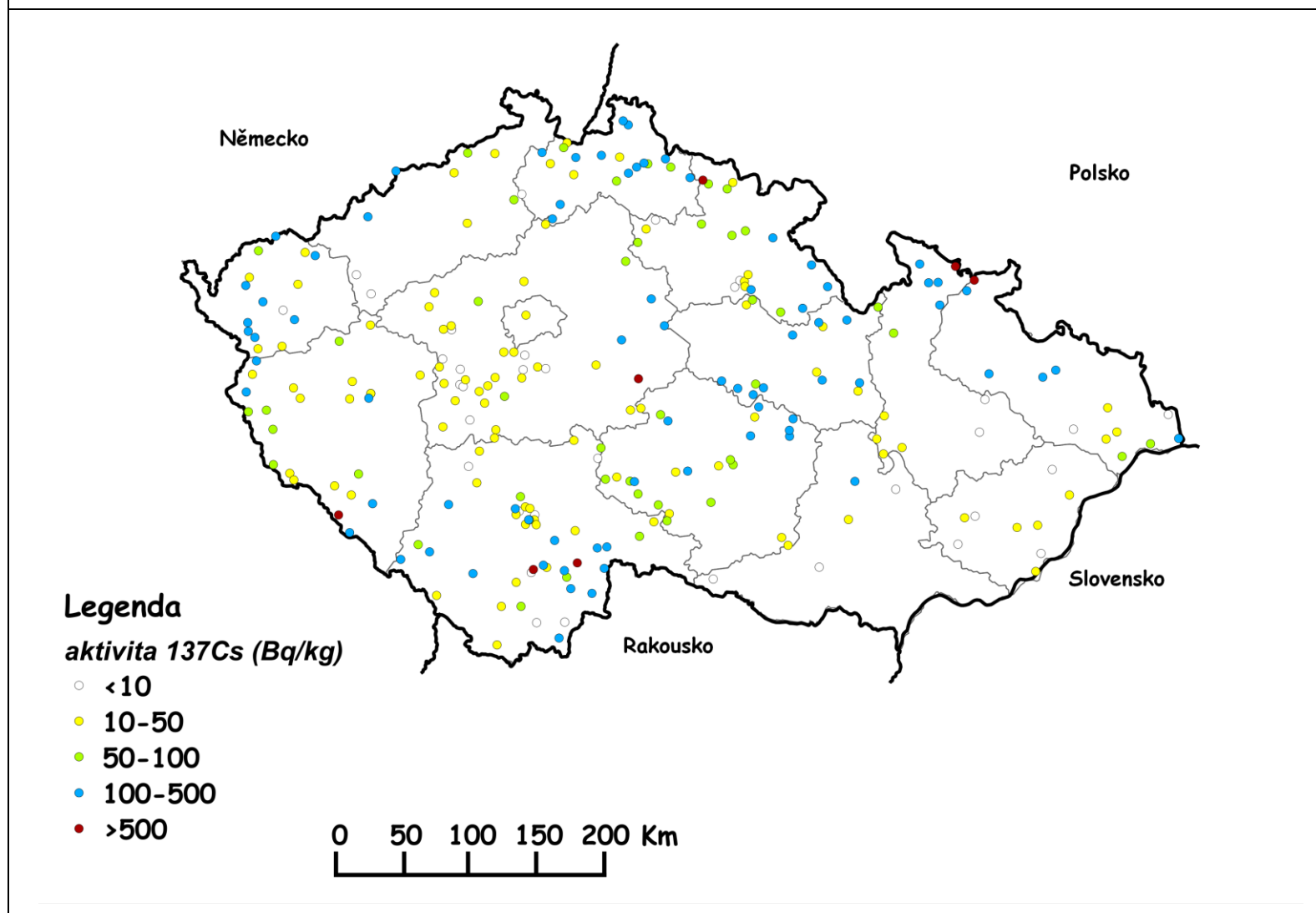
Obr. 1a Hmotnostní aktivity ^{137}\text{Cs} v hřibotvarých houbách na území ČR v letech 2004 – 2012 – bodové zobrazení
