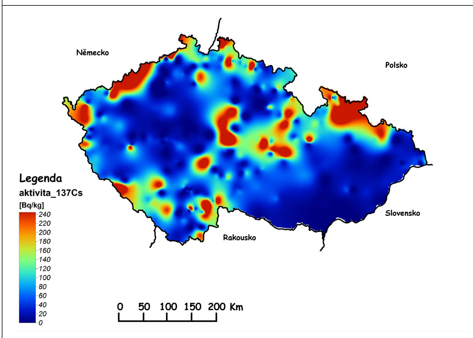
Obr. 2b Hmotnostní aktivity ^{137}\text{Cs} ve všech houbách na území ČR v letech 2004 – 2012 – vyhlazené zobrazení
